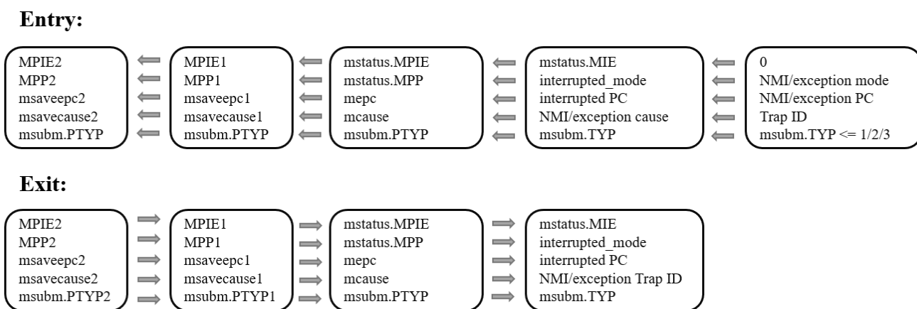
图 4-4 Bumblebee 内核两级 NMI/异常状态堆栈机制示意图
