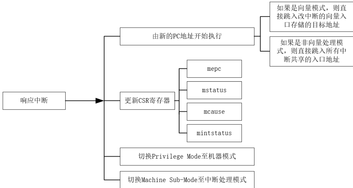
图 5-3 响应中断总体过程
